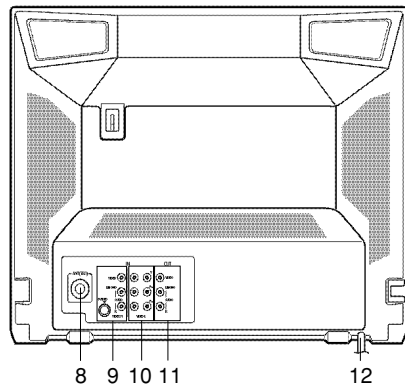
VUE ARRIERE
